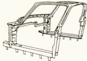
Sport Coupe framework
