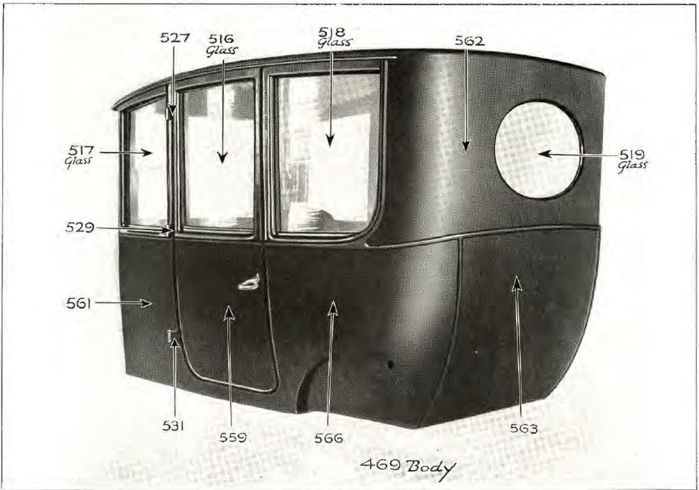
SEDAN BODY
