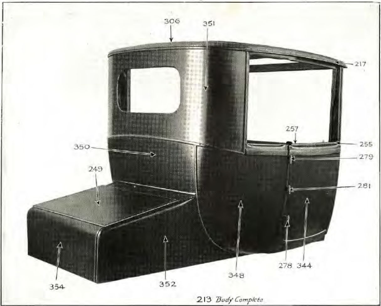
COUPELET BODY
